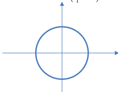
2-范数为1
