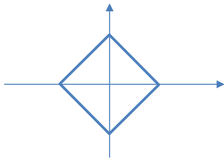
1-范数为1
