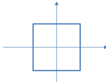
无穷范数为1
